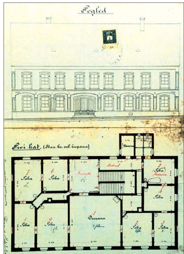
Nacrt zgrade na Trgu Eugena Kvaternika 6. iz 1911. godine (HR DABJ 291 — Zbirka nacrti i planova, Inv. br.A-19).
