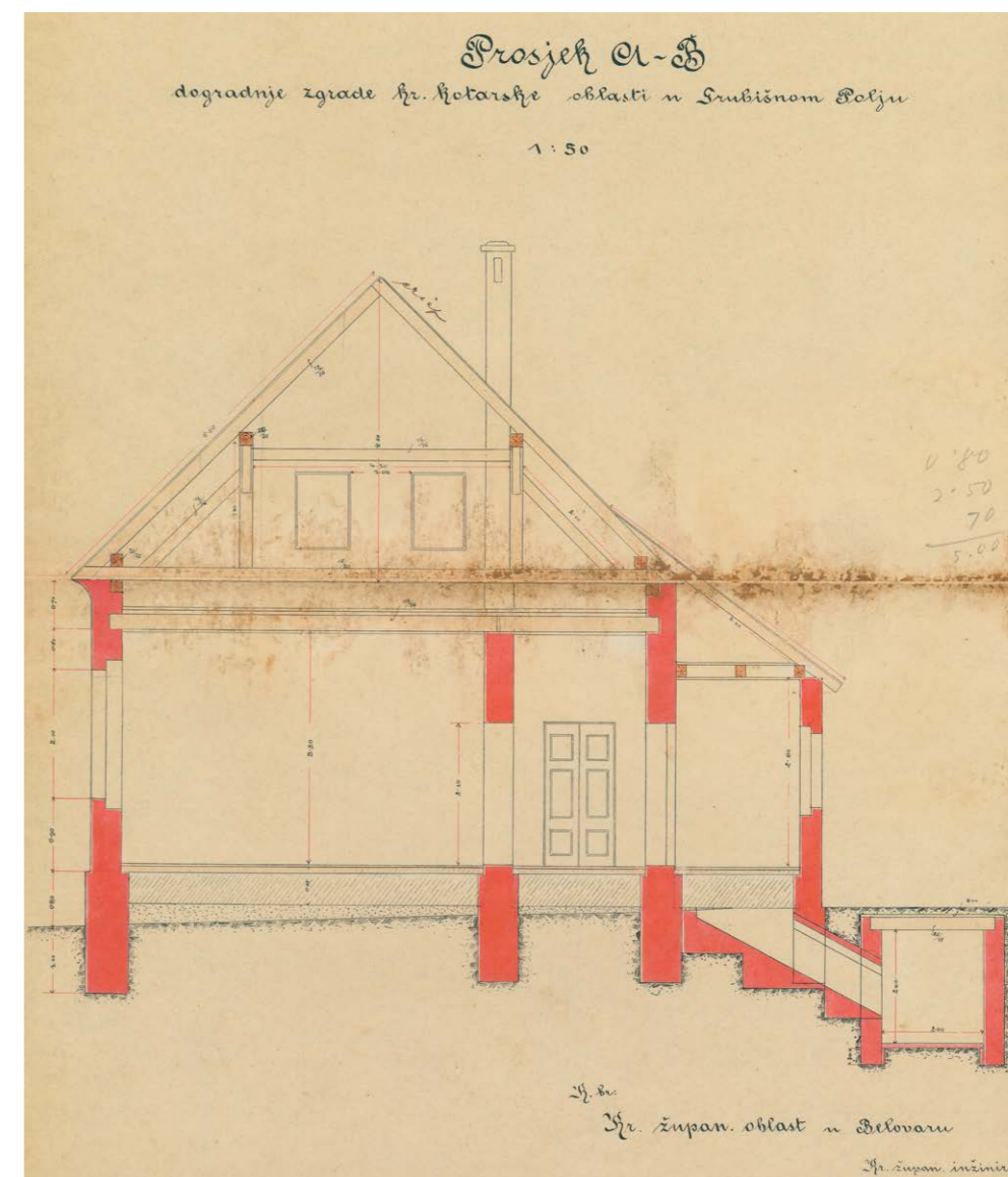
..... Kraljevska kotarska oblast u Grubišnom Polju; nacrt za dogradnju zgrade (presjek) 1897. godina
